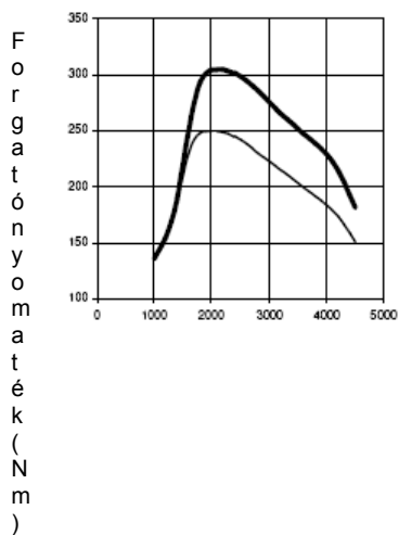
Fordulatszám (fordulat/perc)
