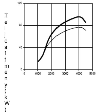
Fordulatszám (fordulat/perc)
