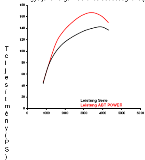
Fordulatszám (fordulat/perc)
