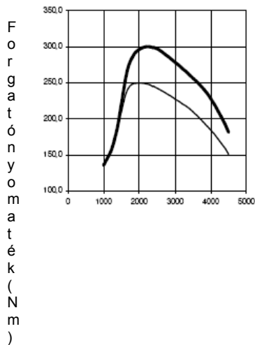
Fordulatszám (fordulat/perc)
