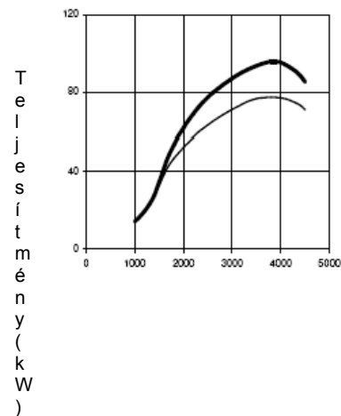
Fordulatszám (fordulat/perc)
