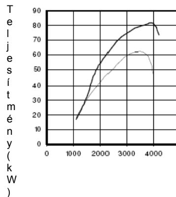
Fordulatszám (fordulat/perc)
