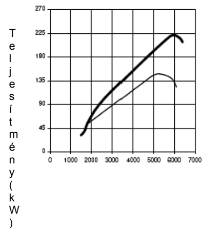
Fordulatszám (fordulat/perc)
