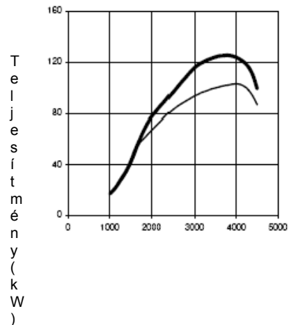
Fordulatszám (fordulat/perc)
