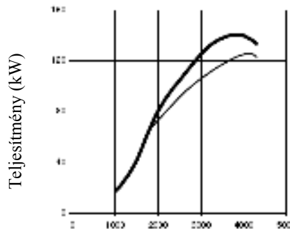
Fordulatszám (fordulat/perc)
